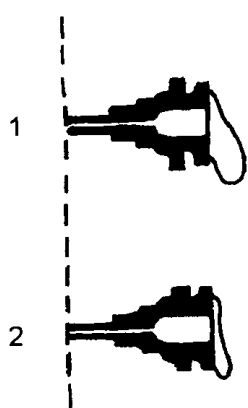
图 1-1-2-5A 悬滴试验
