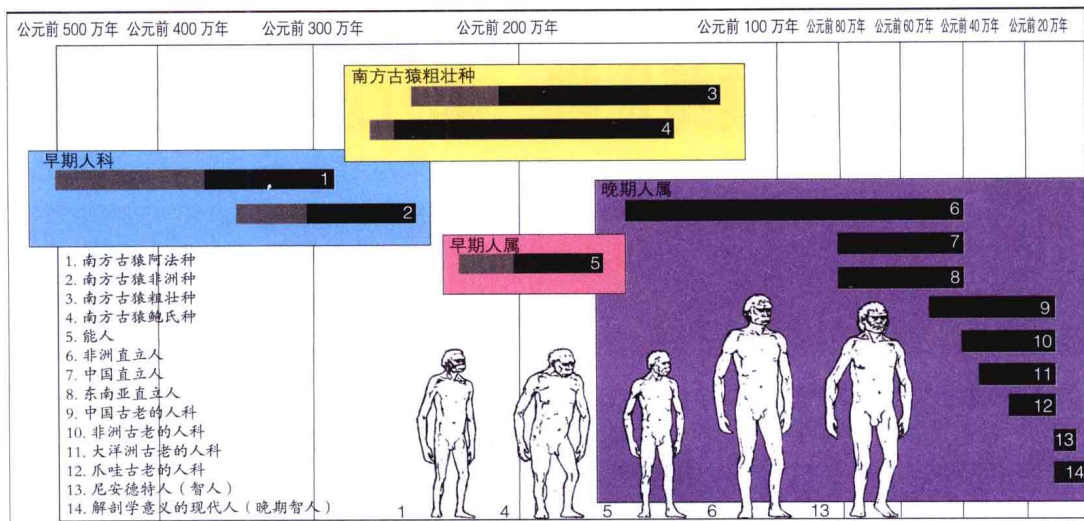
7 人类起源示意图
