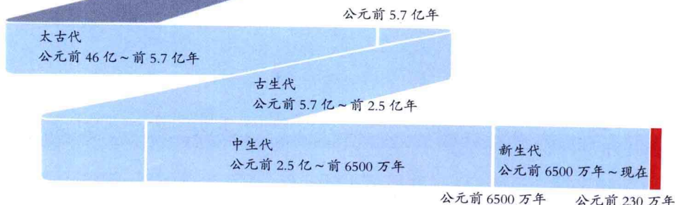
地球年代划分示意图
