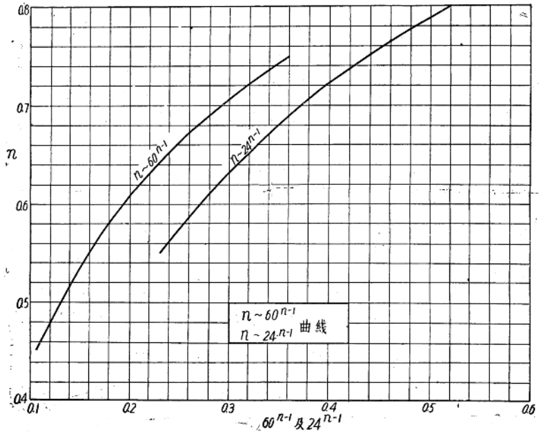
图 32 系数 n 曲线图
