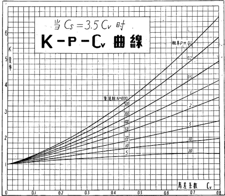
图 30 当 C_s = 3.5 C_v 时, K-P- C_v 曲线
