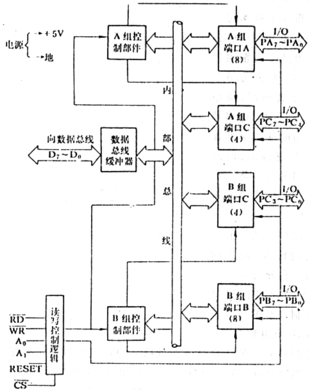
图 1.4 8255 组成
