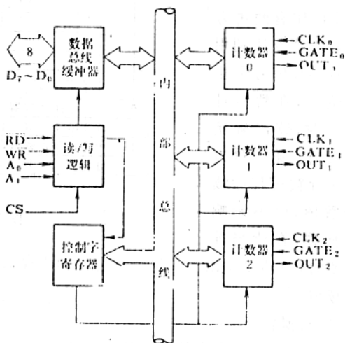
图 1.6 8253 组成
