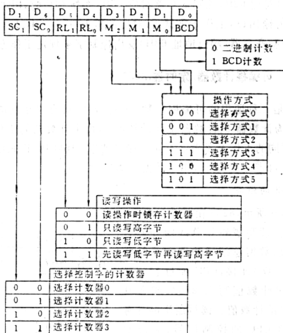
图 1.7 8253 命令字格式
