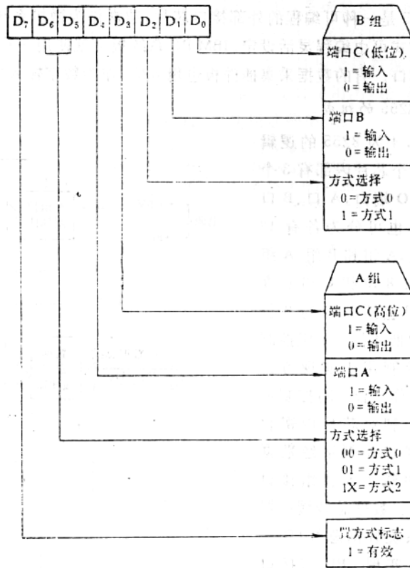
图 1.5 方式命令字格式
