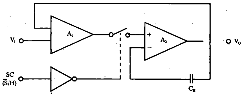
图1 采样/保持放大器结构原理图
