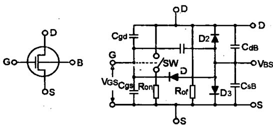
图 2 MOS 开关等效电路
