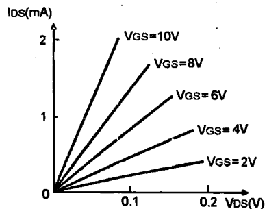
图 3 MOS 管线性电阻区特性曲线
