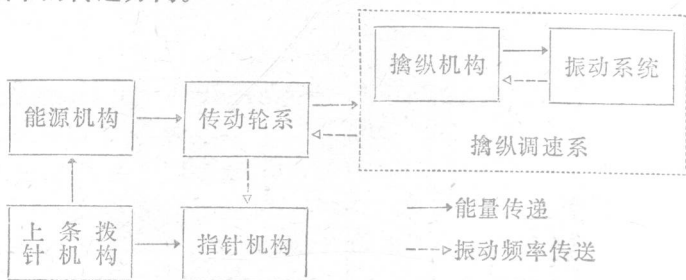
图 1—1 工作原理图
