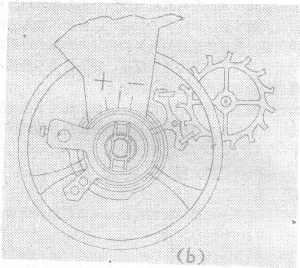
图 1—5 擒纵调速系
