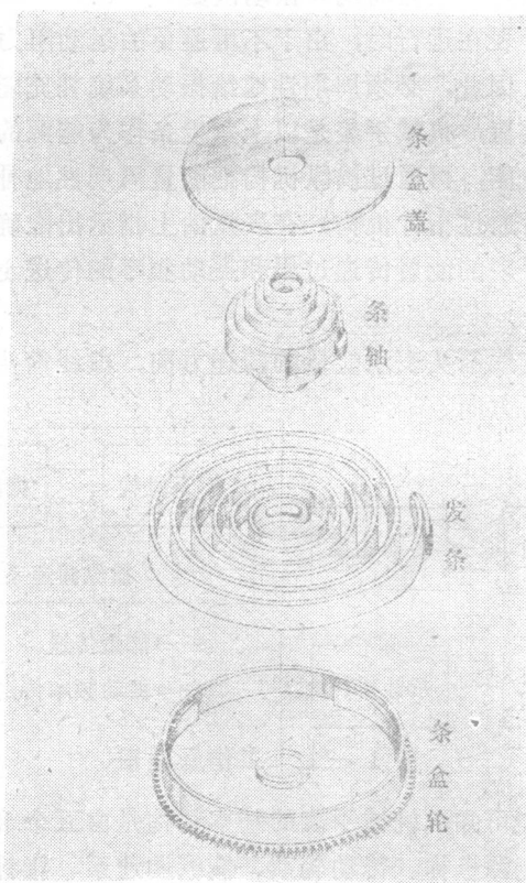
图 1—3 能源机构
