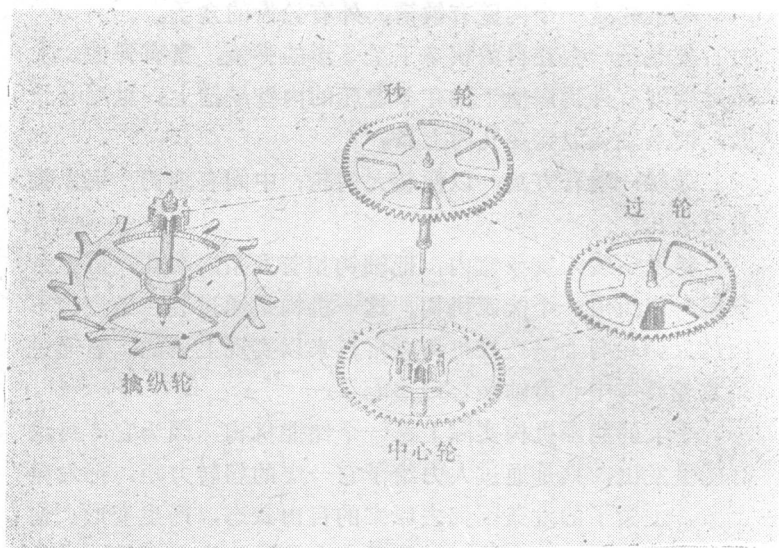
图 1—4 传动轮系
