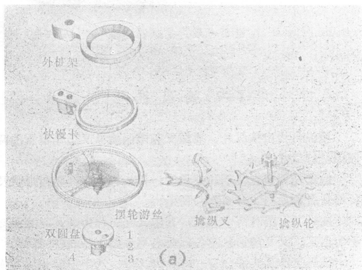
图1—5 擒纵调速系
