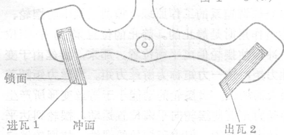
图 1—6 (b) 擒纵叉
