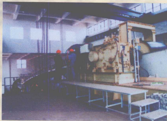
由英国、美国、德国共同设计生产的长2700米的长距离强力胶带机已在成庄矿投入使用
