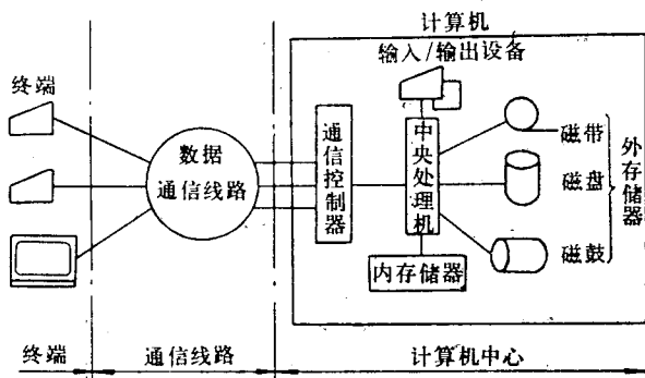
图 1-6 数据通信系统的基本构成
