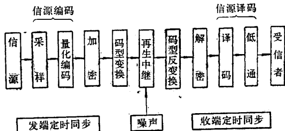
图 1-5 PCM数字电话通信系统
