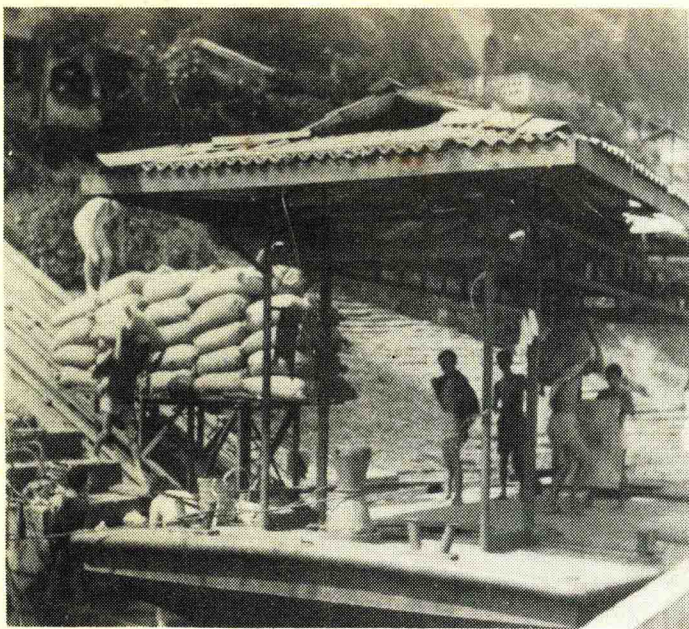
安居码头供装 卸的钢质囤船
