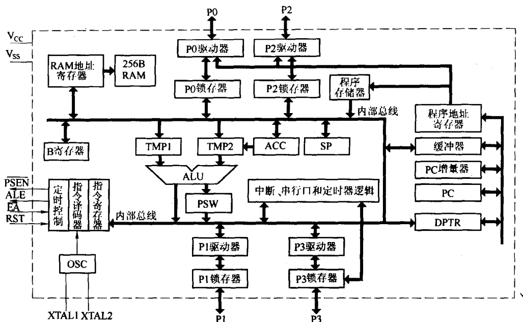
图 1.1 MCS-51 单片机的内部结构
