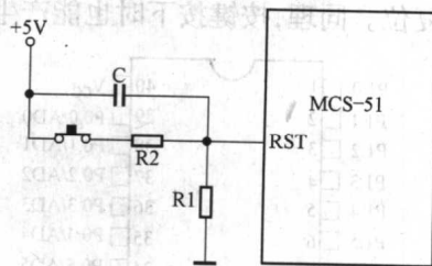
图 1.3 上电/手动复位电路
