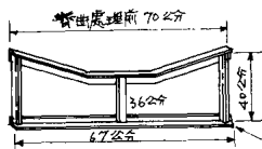
正立面
