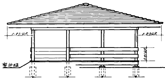
側立面
