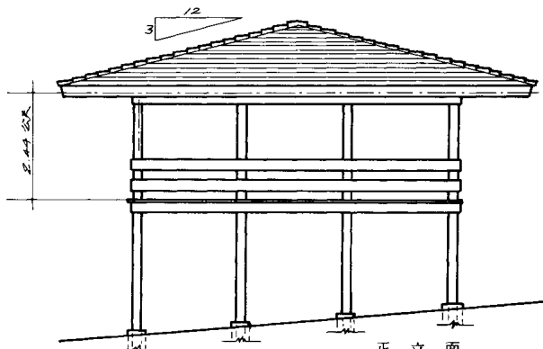
正立面
