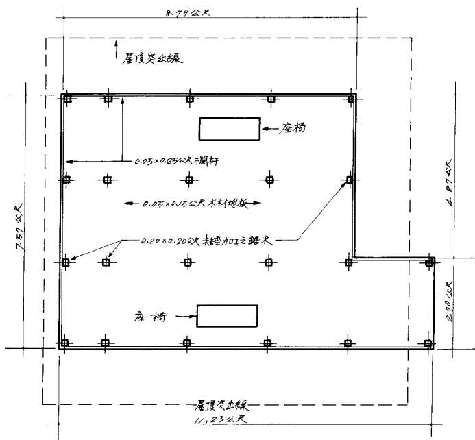
地板平面
