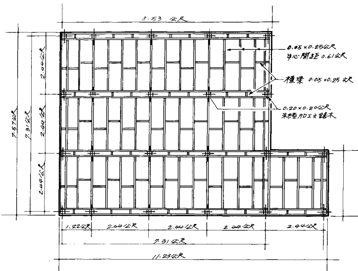
地板架構平面圖
