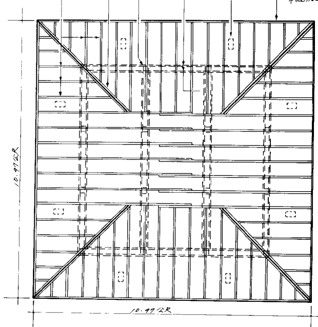
屋頂構架平面
