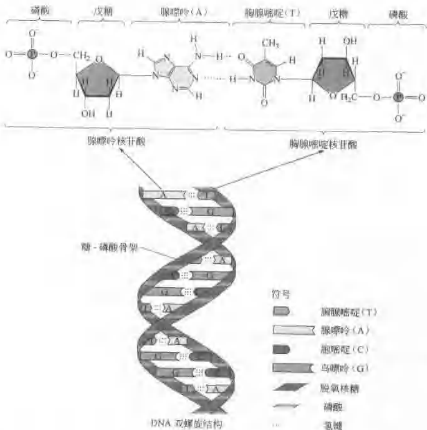
图 2-1 DNA 的组成
