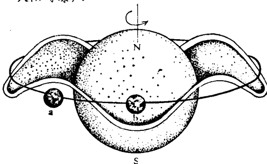
太阳与暴风
