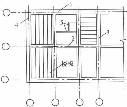
图 1-2 墙的类型
