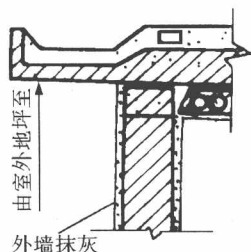
图 1-3 外墙抹灰计算高度示意图(有挑檐天沟)
