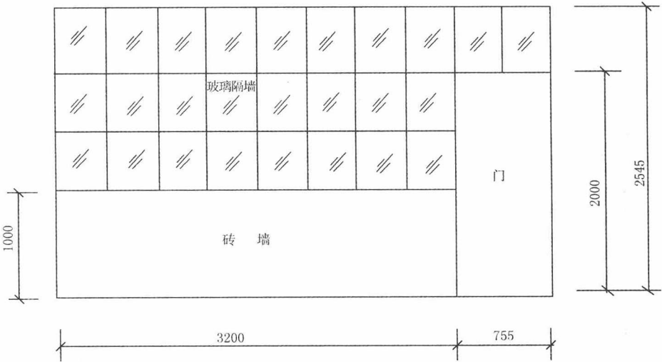
图 1-9 玻璃隔墙示意图
