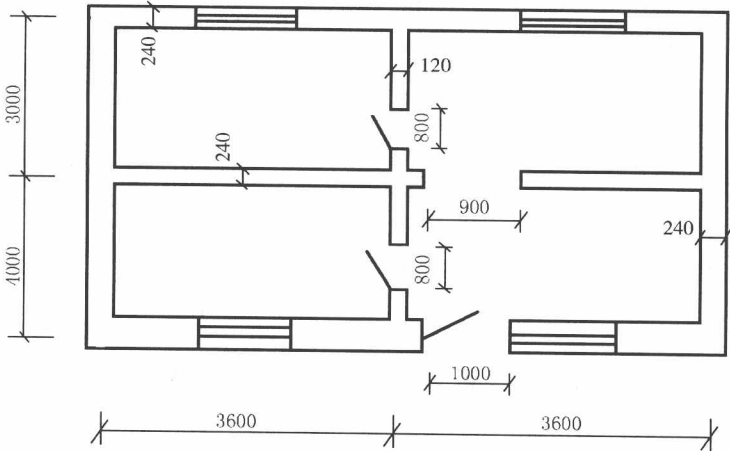
图 1-6 某房间示意图
