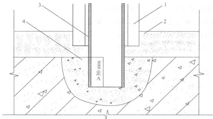
图 1-1 预留洞法拼墙料与墙体的固定
