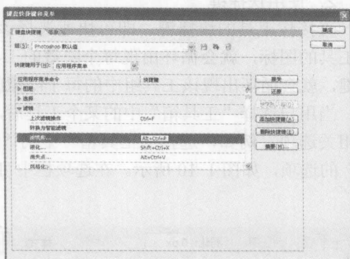
图 1-7 输入快捷键
