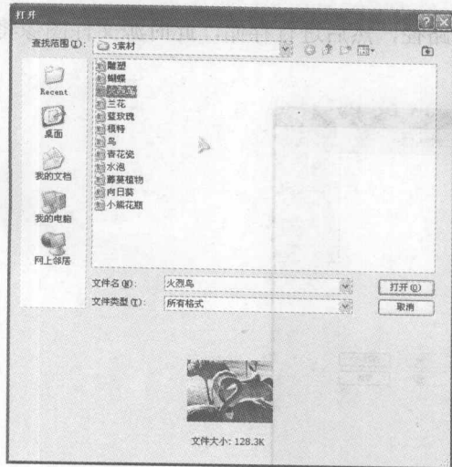
图 1-18 “打开”对话框
