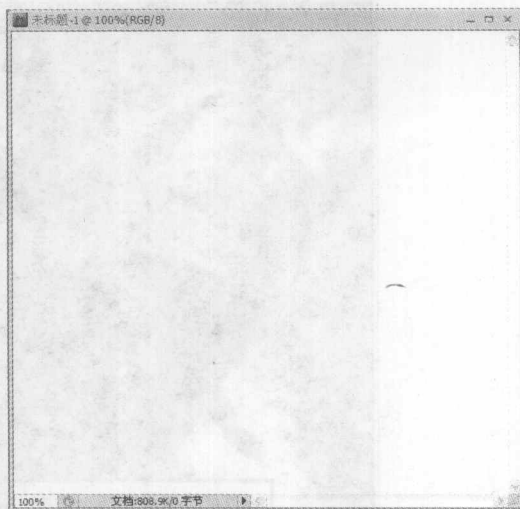
图 1-17 新建图像
