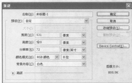
图 1-16 “新建”对话框
