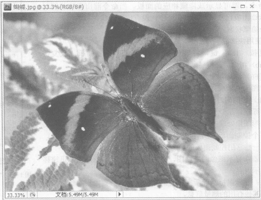
图 1-12 打开图像
