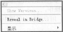
图 1-13 弹出的菜单
