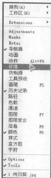
图 1-11 “窗口”菜单
