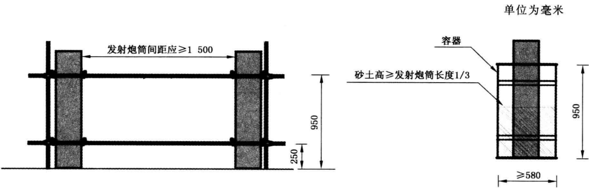
图 B.4 10号以上发射炮筒固定示意图
