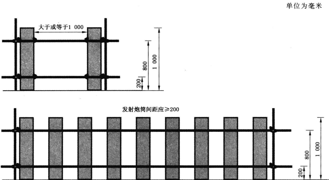
图 B.3 7号、8号发射炮筒固定示意图
