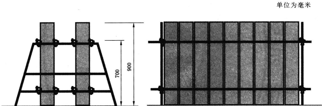
图 B.2 5号、6号发射炮筒固定示意图
