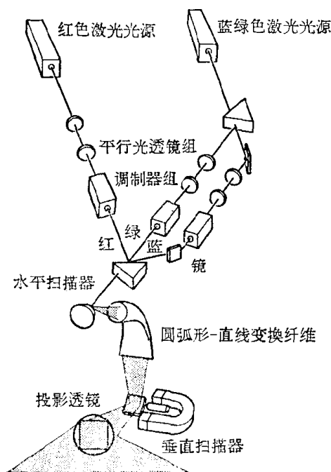
图 2 多色激光显示器
