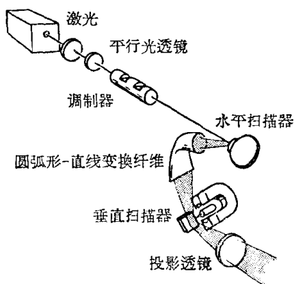
图1 单色激光显示器
