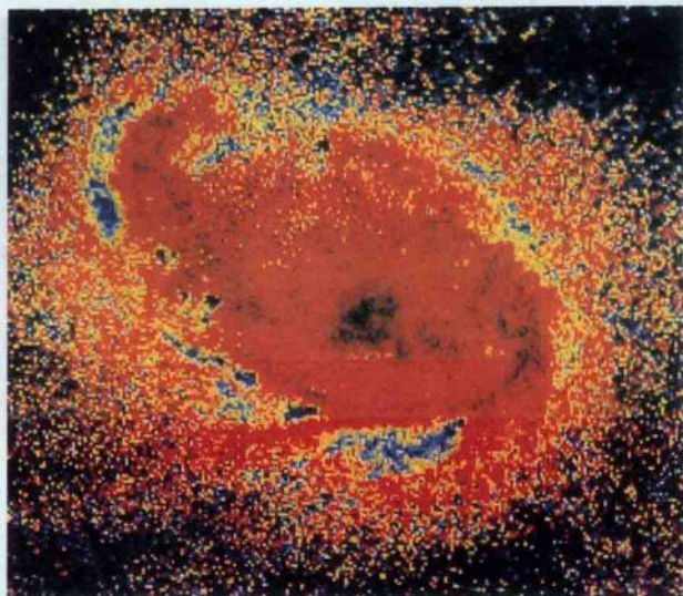
◎ 星际物质在宇宙空间的分布并不均匀，在引力作用下，某些地方的气体和尘埃可能相互吸引而密集起来，形成云雾状。人们形象地把它叫做“星云”
