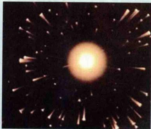
◎ 大爆炸时的宇宙
