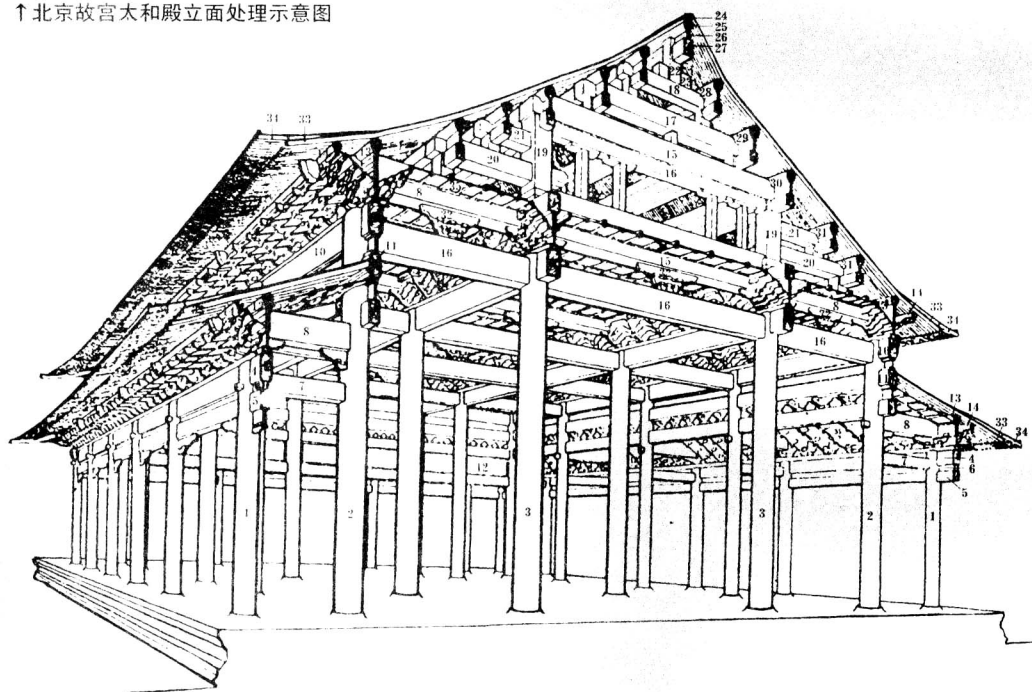
↑ 故宫太和殿梁架结构示意图
