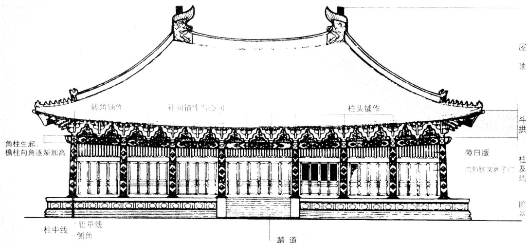
↑ 北京故宫太和殿立面处理示意图
