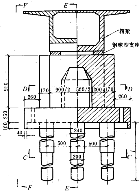
图 1-1-3 主桥桥墩 尺寸单位:cm
