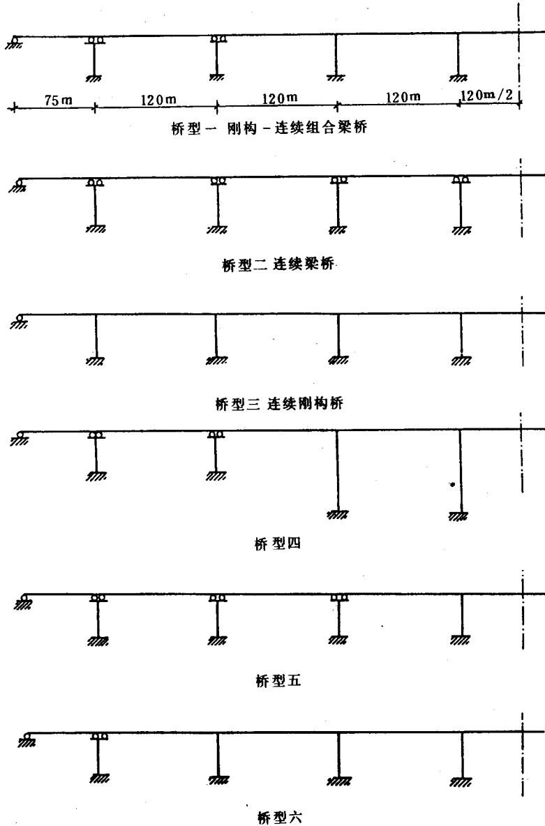
图 1-2-1 进行结构体系分析的各种计算图式
