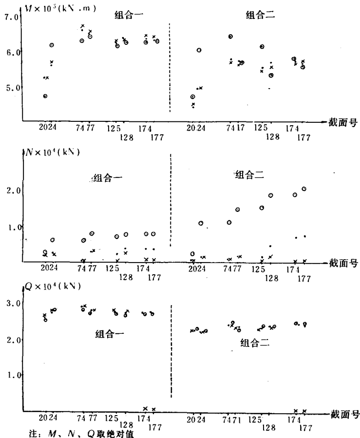
图 1-3-2 桥型一、二、三主梁支点控制截面 M 、 N 、 Q 内力比较
