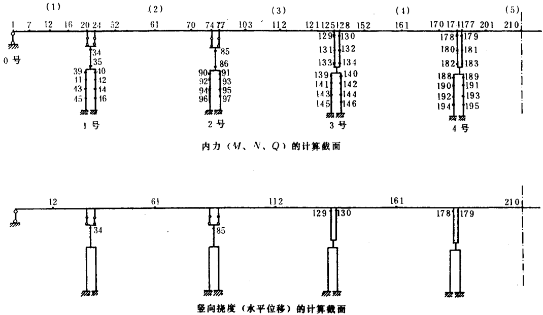
图 1-2-2 内力和位移的计算截面
