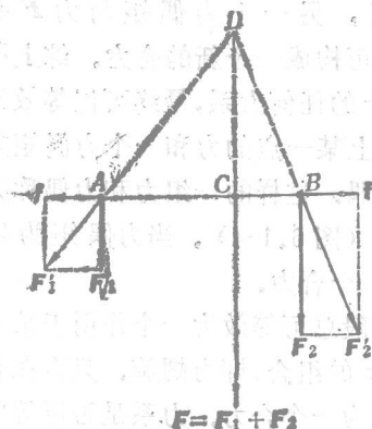
图 6.1-2 求平行力的合力
