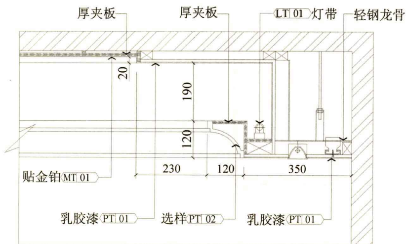
图1.10 住宅空间设计剖面图和大样图 文健、石树勇
