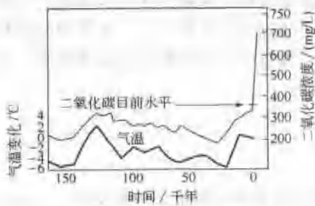
图 1-1 自然状态下二氧化碳随时间浓度变化
