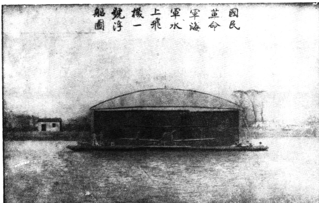
海军飞机工程处建造的水上飞机浮坞
