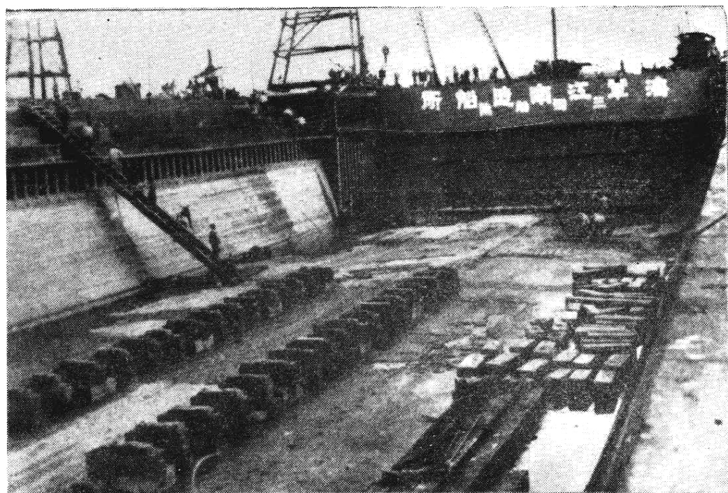
海军江南造船所三号船坞
