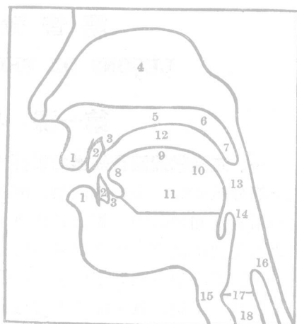
发音器官图
