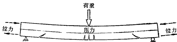
图 1-1 混凝土梁受力示意图
