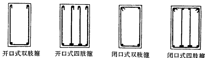
图 1-3 箍筋的构造形式
