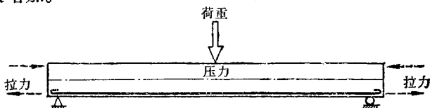
图 1-2 钢筋混凝土梁受力示意
