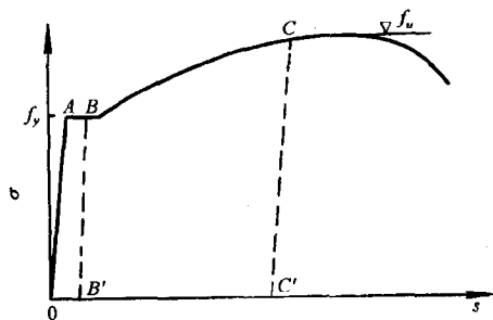
图 1.16 建筑钢材的应变硬化
