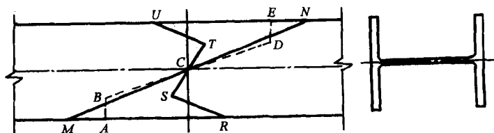
图 1.12 矫直产生的残余应力
