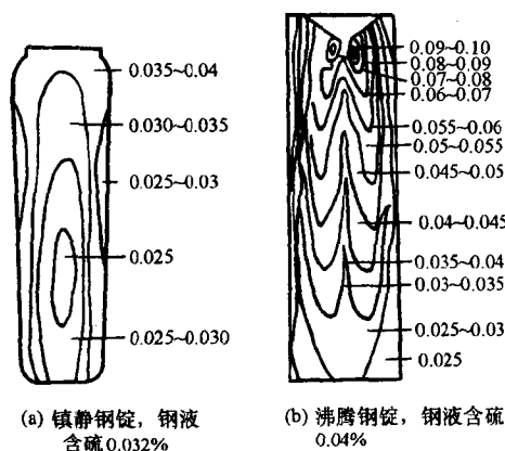
图 1.13 钢锭中硫的偏析
