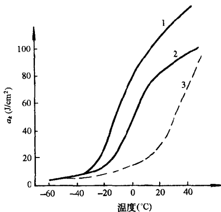
图 1.17 应变硬化使冲击韧性降低
