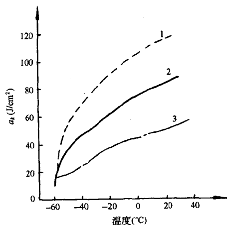
1. 纵向试样; 2. 横向试样; 3. 人工时效后横向试样
