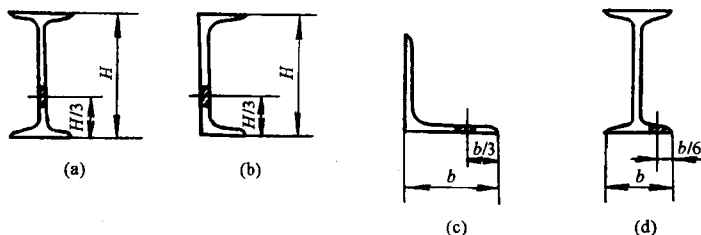
图 1.9 型钢试件取样
