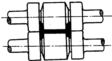
图 1.8 工字钢轧辊
