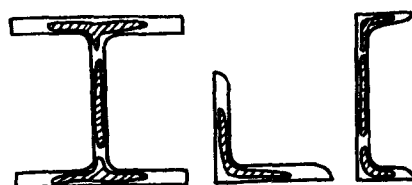
图 1.14 型钢硫的偏析
