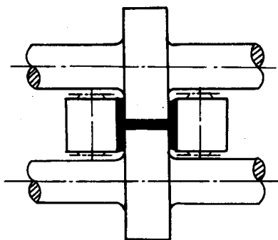
图 1.10 宽翼缘工字钢轧制
