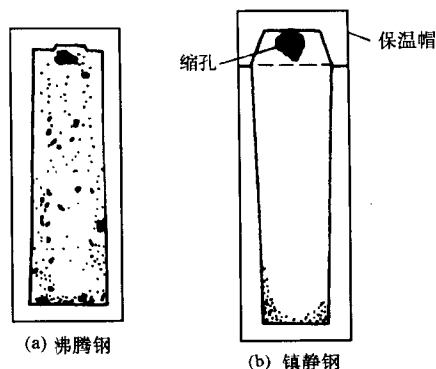
图 1.3 钢锭剖面
