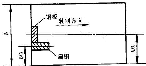
图 1.7 钢板和扁钢试样取样
