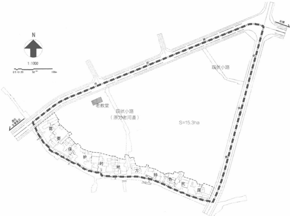
图1-4 江南某风景旅游城镇入口地段规划设计
