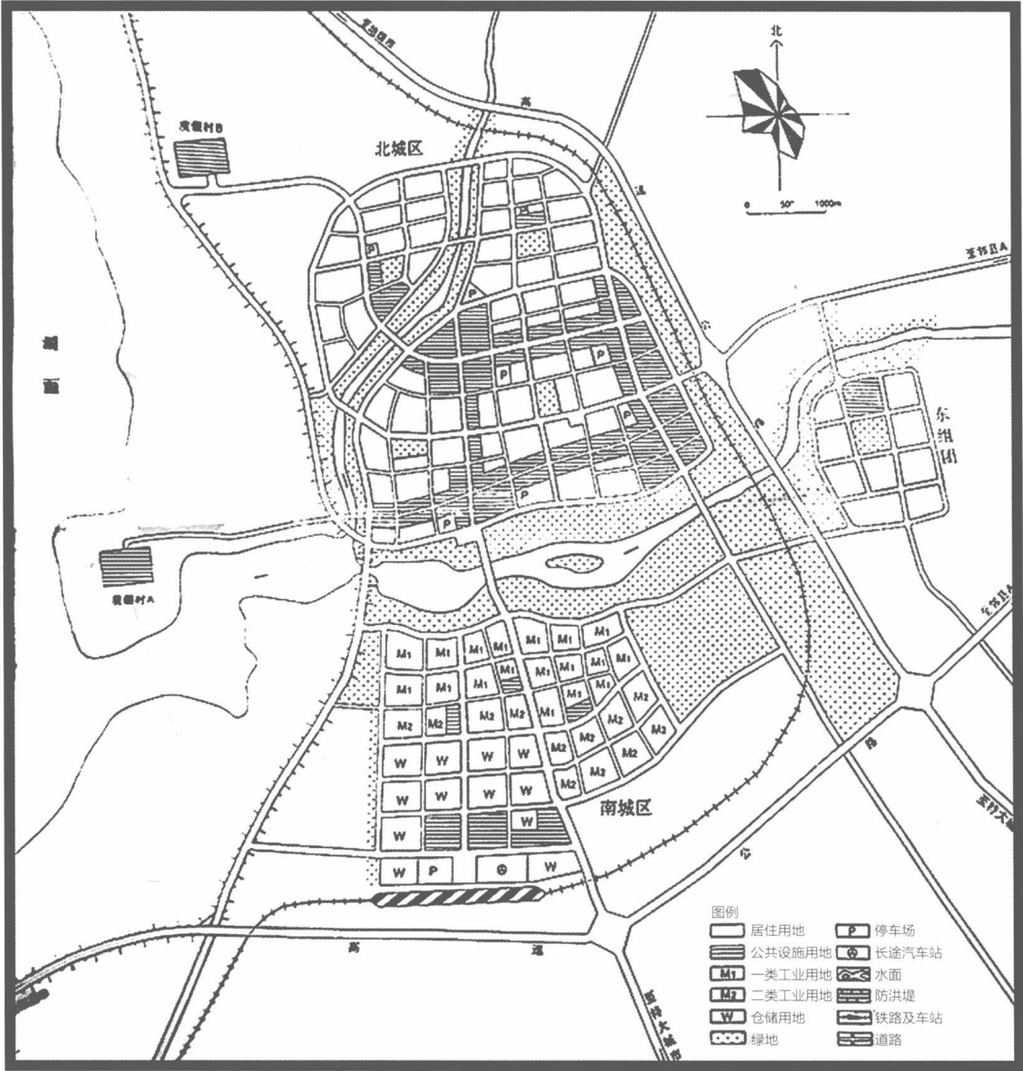
图1-1 某城市主城区总体规划方案
