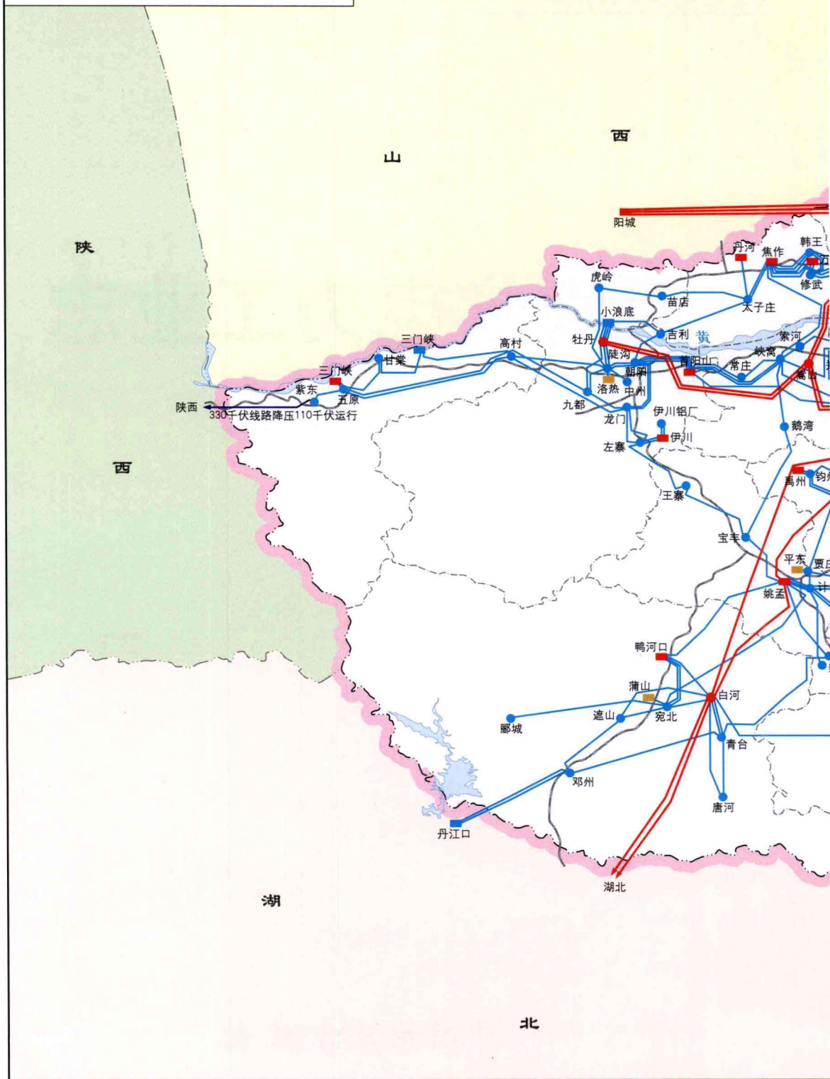
2002年河南省电网地理接线示意图
