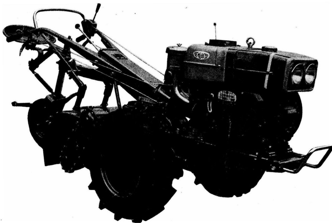
地产清水江—1型手扶拖拉机
