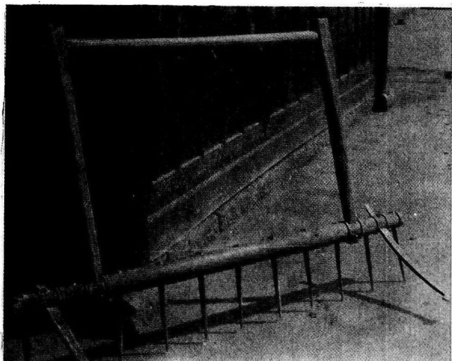
手 耙
