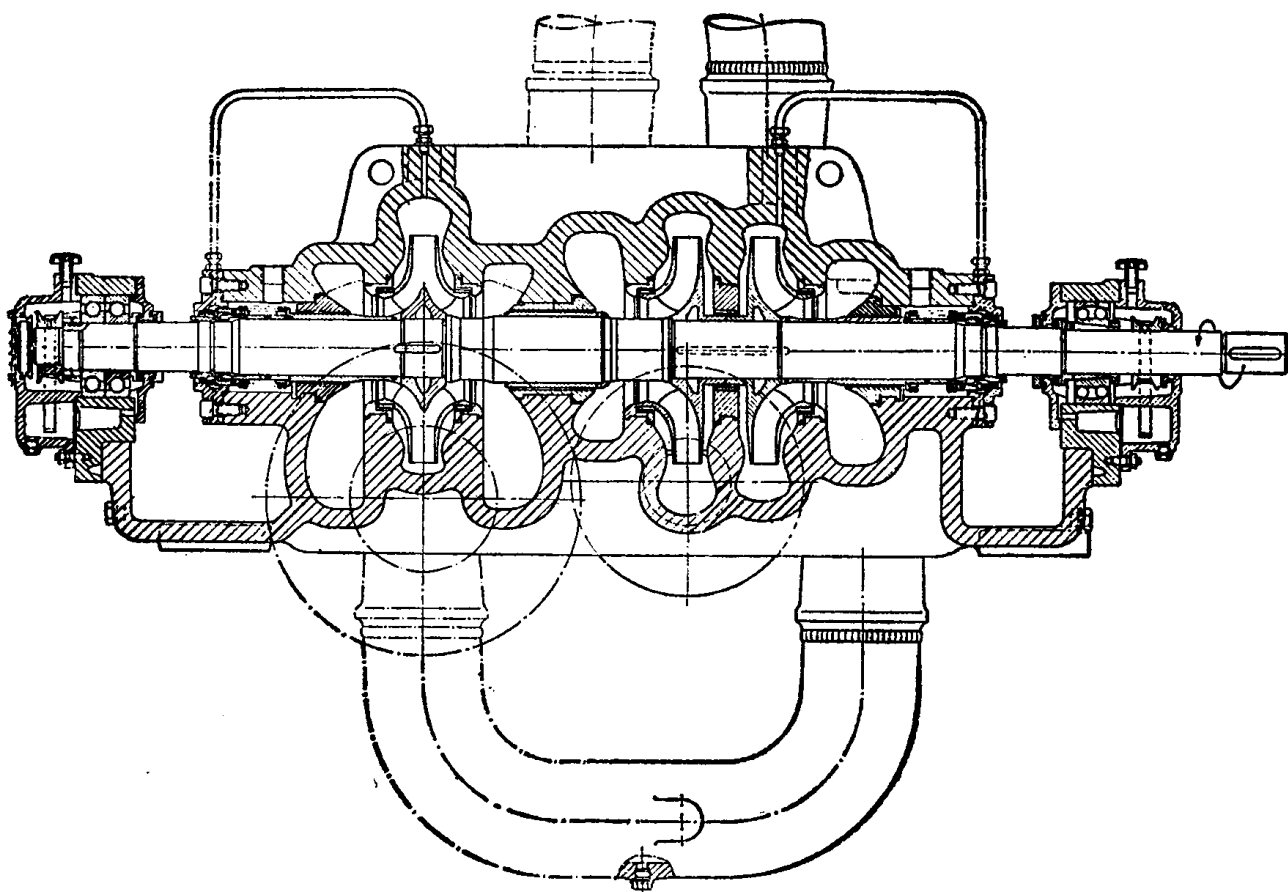
图 1-7 蜗壳式多级泵
