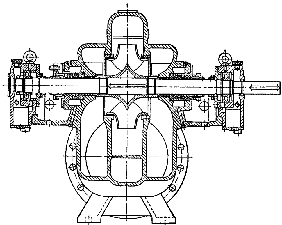
图 1-6 单级双吸泵
