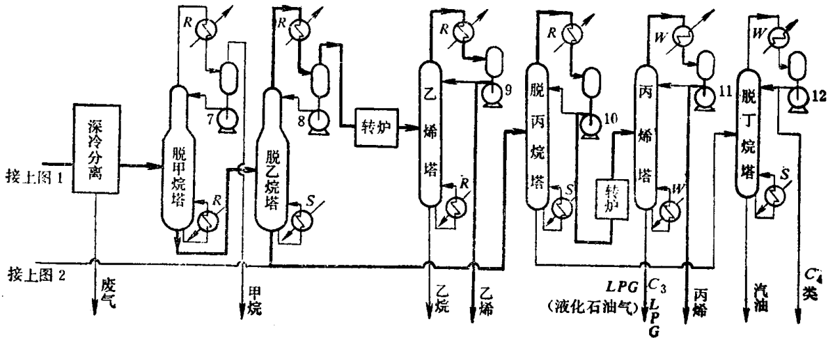
图 1-14 化工流程 (乙烯装置)
