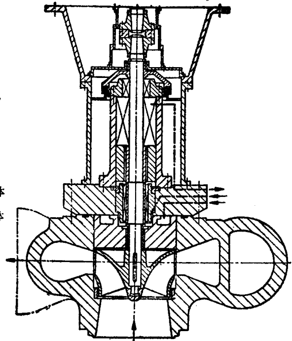
图 1-13 压水式反应堆系统冷却泵
