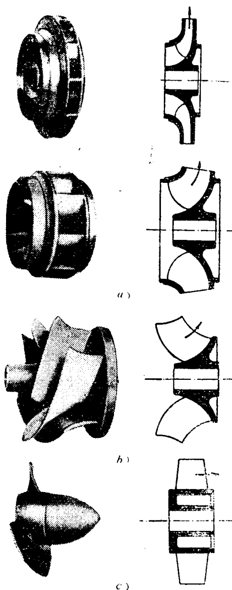
图1-4 叶轮的类型
