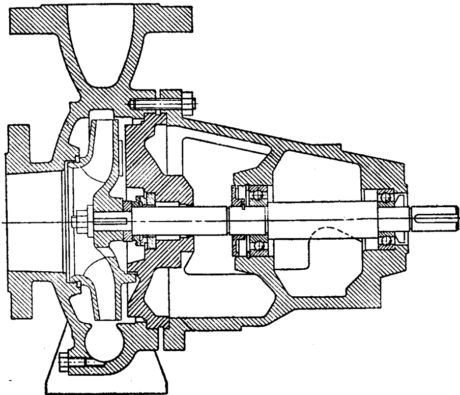
图 1-5 单级悬臂式泵
