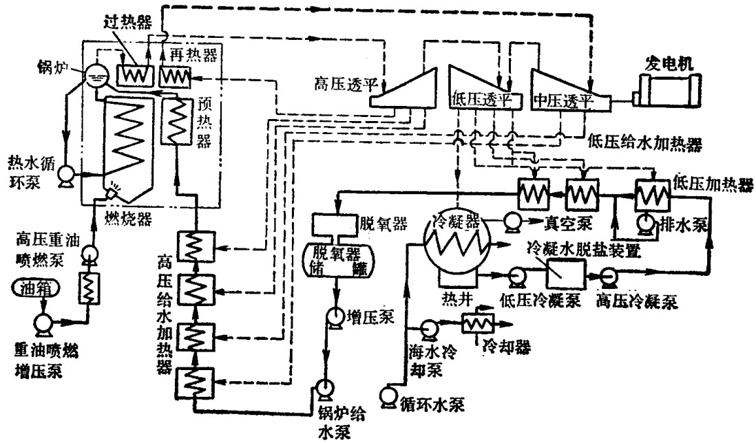
图 1-10 热电厂主要水汽系统图
