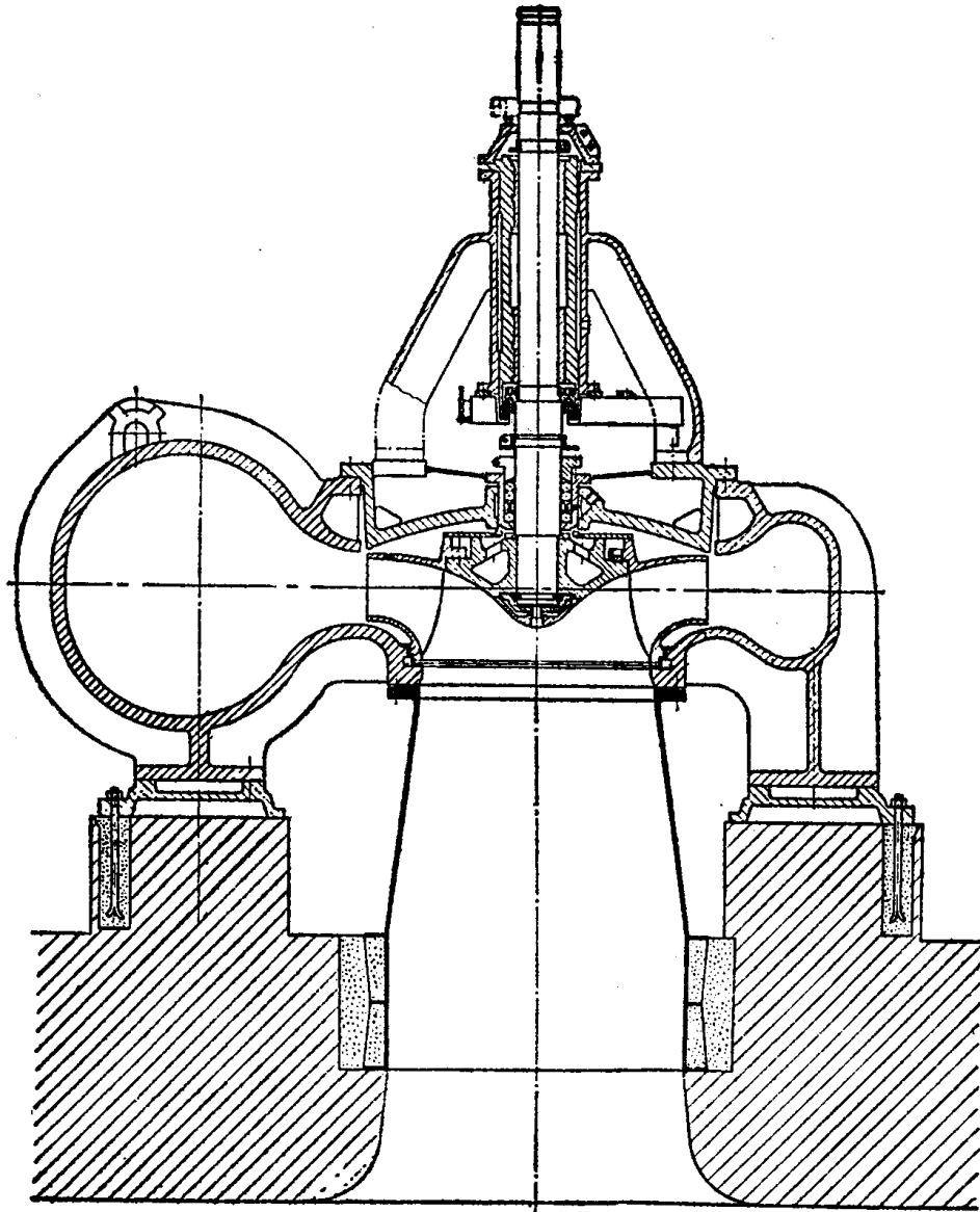
图 1-9 大型单级立式泵
