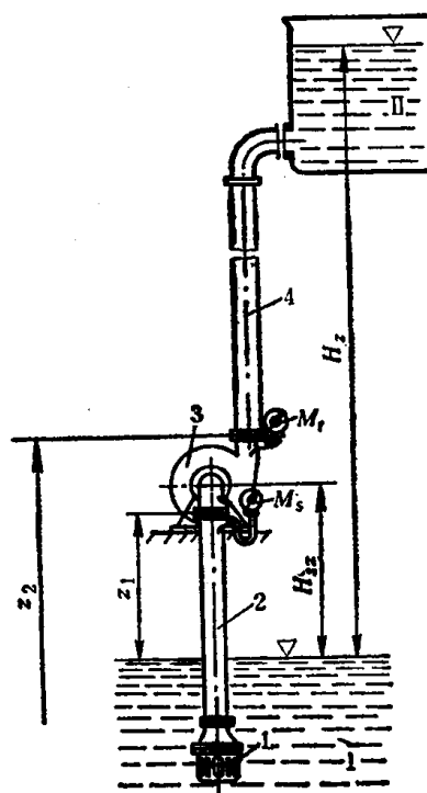
图 1-1 泵装置简图
