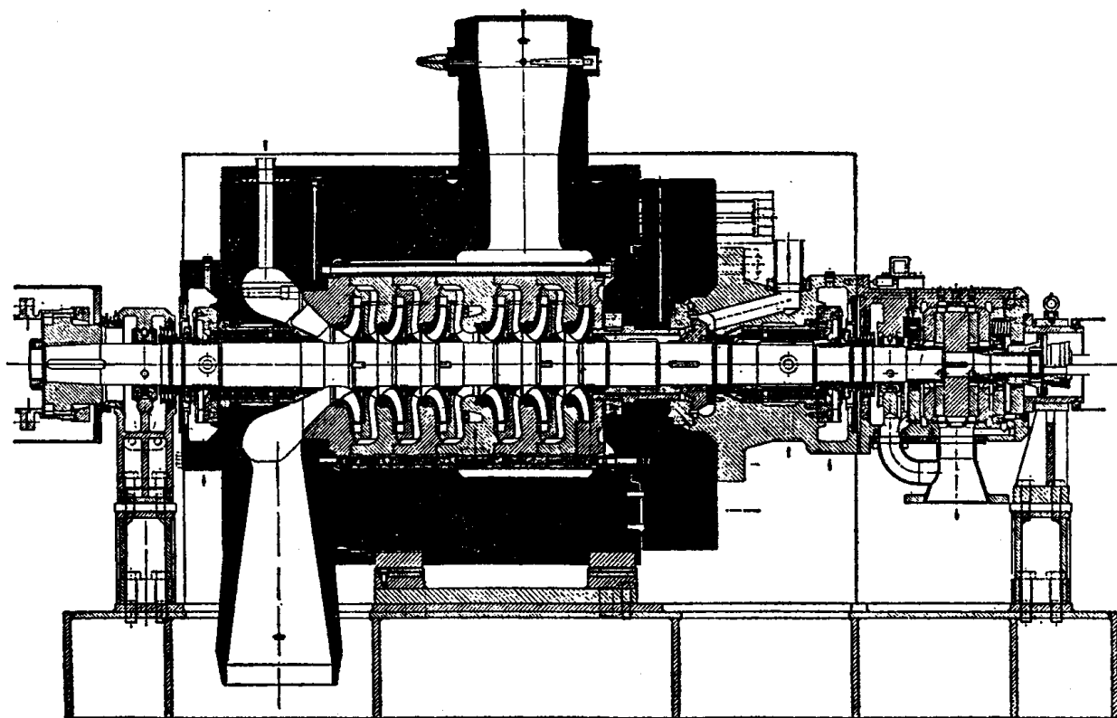
图 1-11 近代高温高压锅炉给水泵
