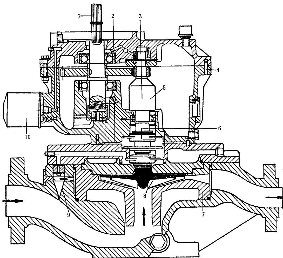
图 1-15 化工流程高速离心泵
