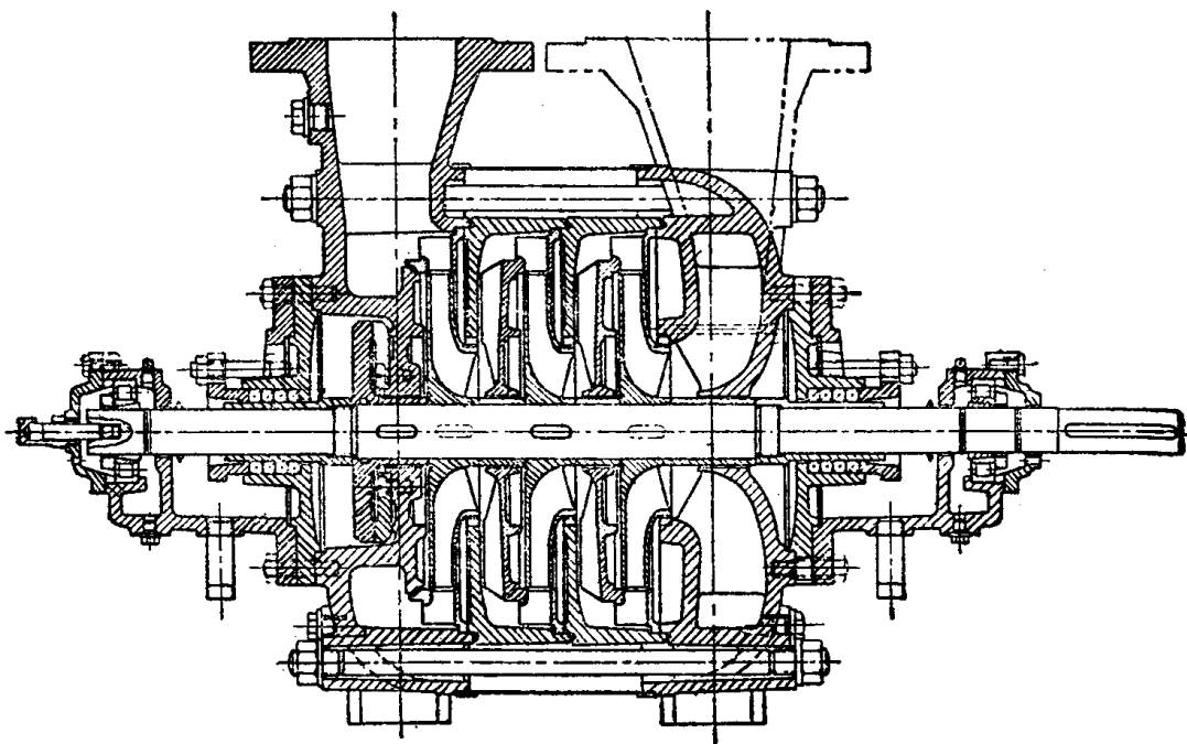
图1-8 节段式多级泵
