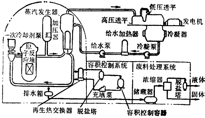
图 1-12 压水式反应堆系统
