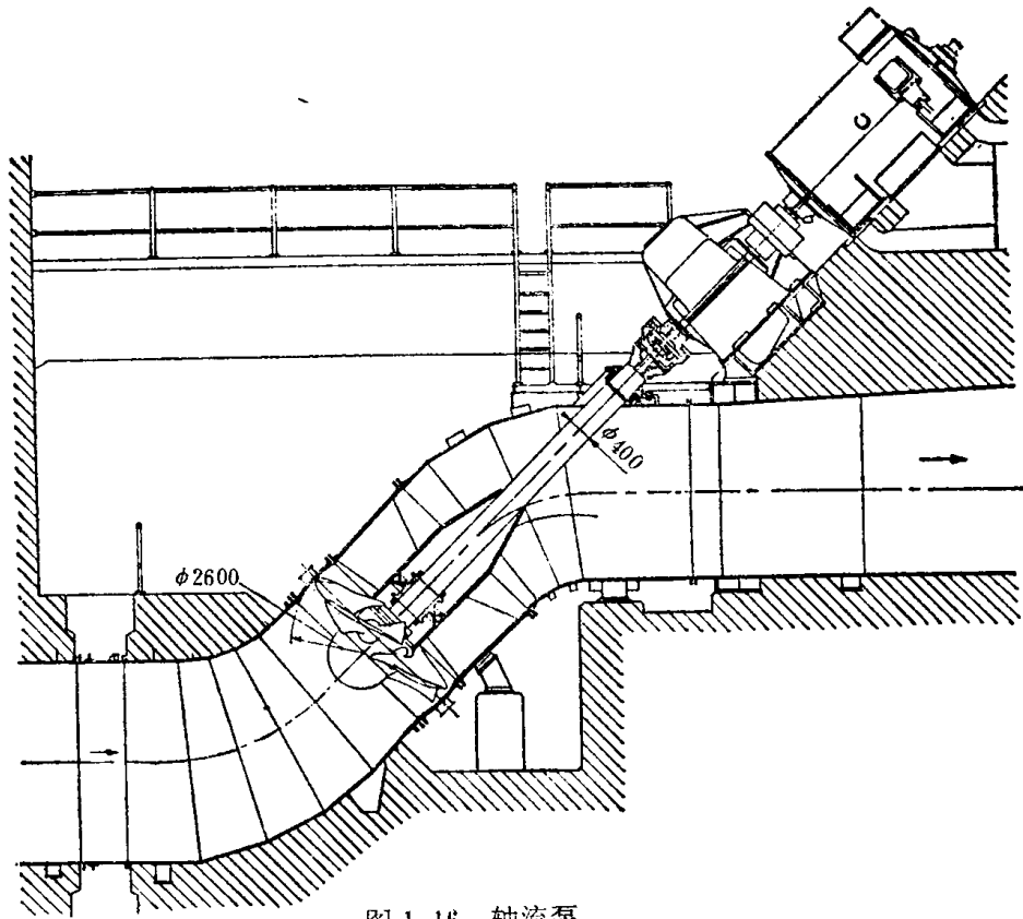
图 1-16 轴流泵
