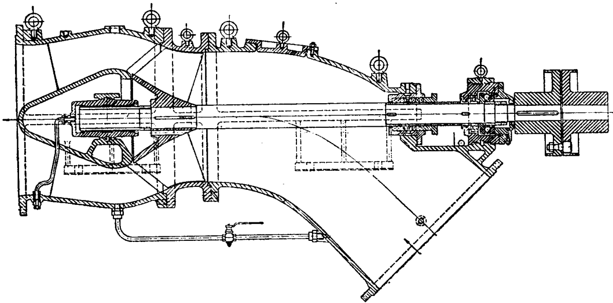
图 1-17 导叶式混流泵
