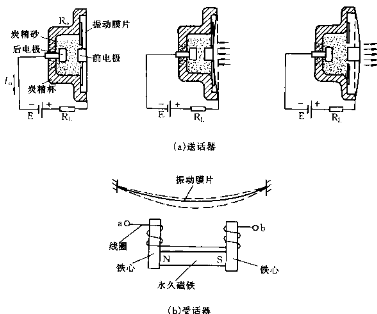
图 1-3 送话器、受话器的构成原理
