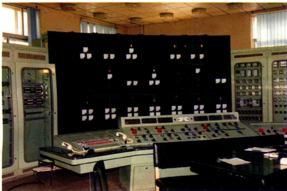
发电厂中央控制室
