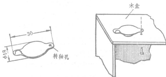
图 1-6 小 盖 片
