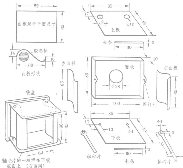
图 1-3 铁 盒
