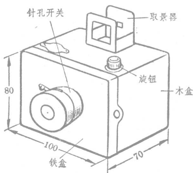
图 1-2 针孔照相机外形
