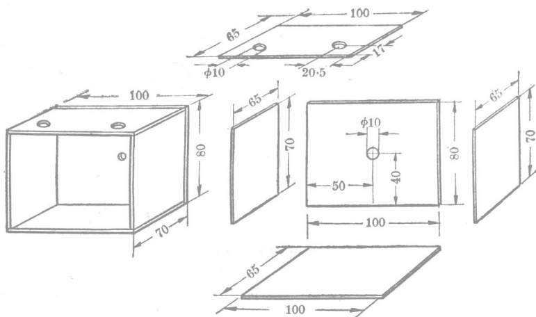
图 1-4 木盒(设计板厚 5 毫米)
