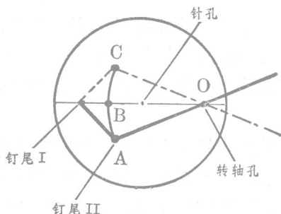
图 1-8 开关原理
