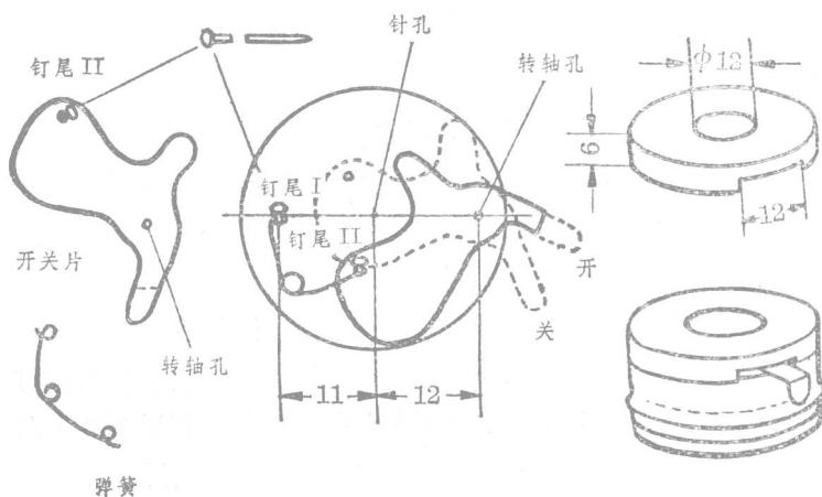
图 1-7 针孔开关(比例 1:1)
