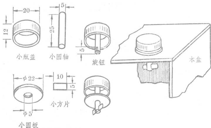
图 1-5 旋 钮
