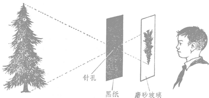
图 1-1 针孔成像
