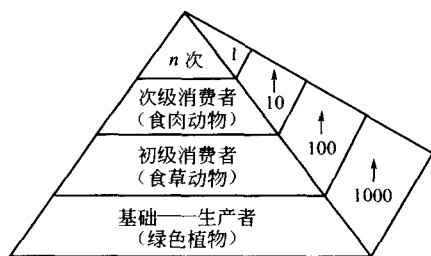
图 1-1 能量传递的 1/10 律 (祝延成等, 1993)
