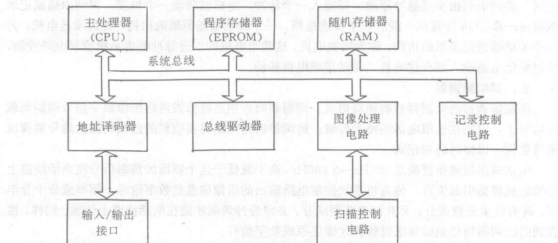
图 1-2 主控电路方框图
