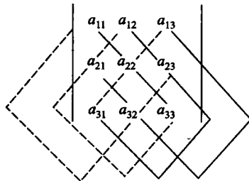
图 1.1 三阶行列式的对角线法则
