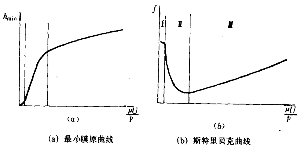
图 1-1 润滑状态
