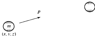
图 1-1 粒子的运动
