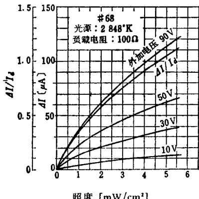
图 5-9 PbS 光敏电阻的照度-输出电流和灵敏度特性
