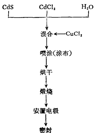
图 5·5 烧结型 CdS 光敏电阻的制造工艺
