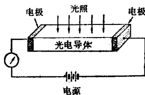
图 5.1 光敏电阻
