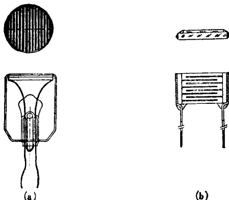
图 5-8 多晶型 CdS 光敏电阻(烧结法)
