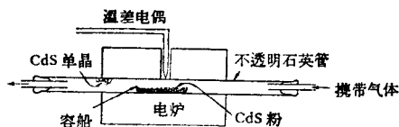
图 5.4 CdS 单晶的制造装置(升华法)
