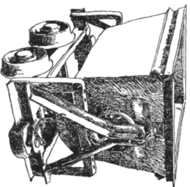
0.55—0.75立方米翻斗式小矿车
