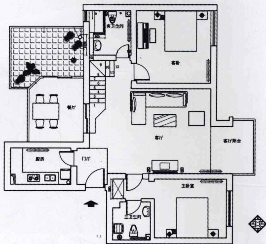
平面布置图
