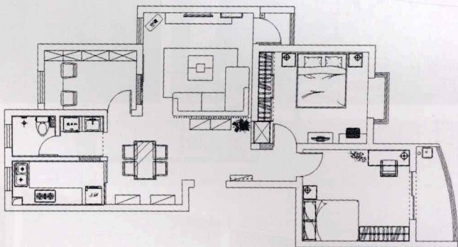
平面布置图
