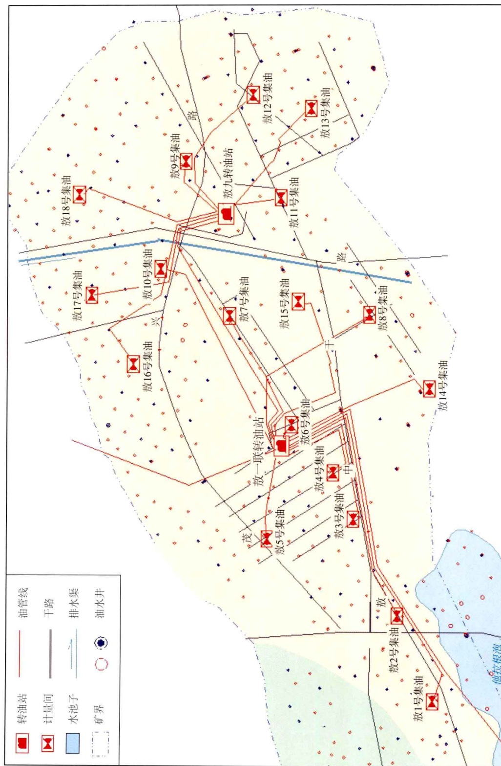
敖包塔油田地面生产系统平面图 (资料来自大庆油田有限责任公司第七采油厂, 2005 年)
