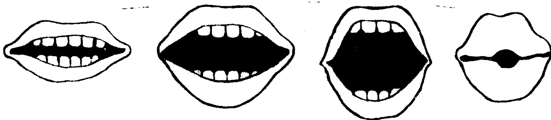
图3 非圆唇音、中度唇音、开圆唇音和闭圆唇音的发音示意图
