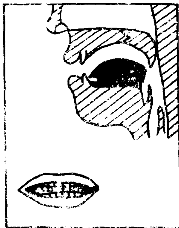
图10 [ə]发音示意图
