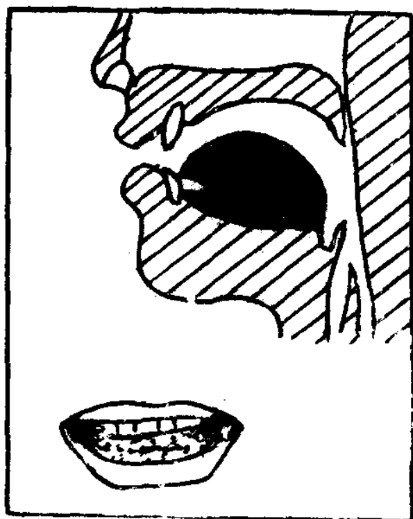
图 6 [e]发音示意图
