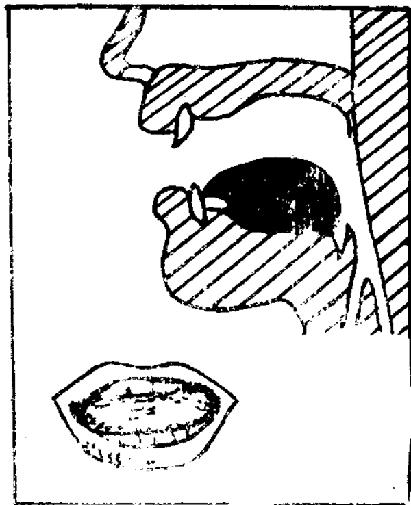
图7 [æ]发音示意图
