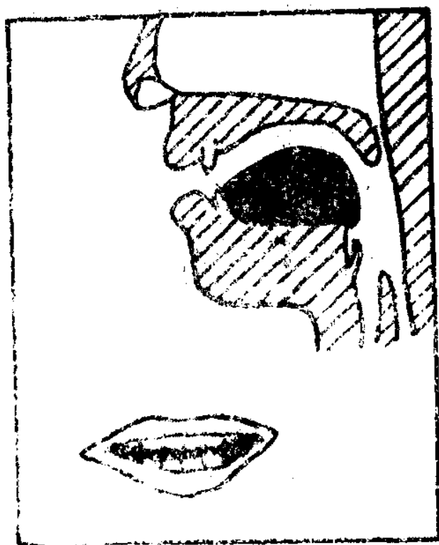
图9 [ə:]发音示意图
