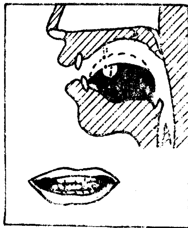
图5 [i]发音示意图
