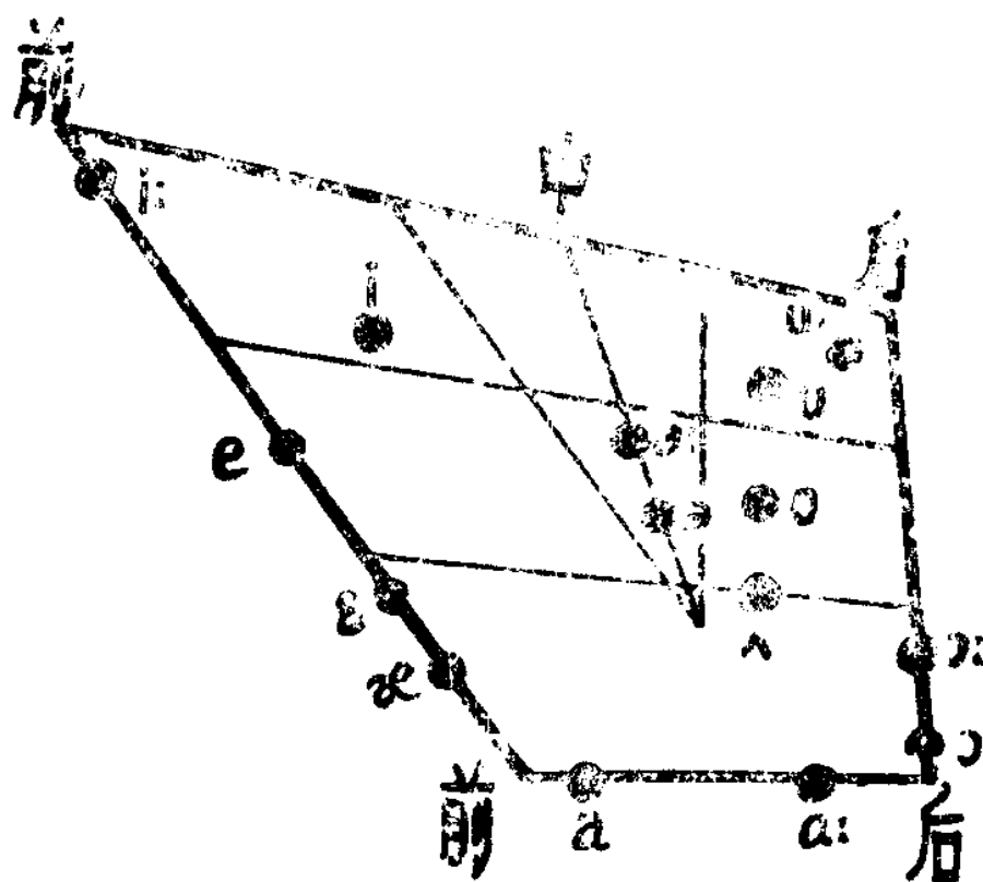
图2 单元音舌位图
