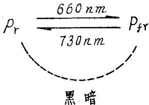
图1 光敏色素Pr与Pfr之间相互转换的关系
