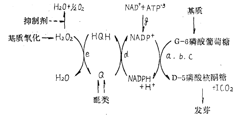
图3 关于发芽过程中G—6—磷酸葡萄糖代谢的设想示意图(按Hendrick等1975) a: D—6—磷酸葡萄糖, DADP+1—氧化还原酶。 b: 6—磷酸葡萄糖酸内酯脱氢酶。 c: 6—磷酸葡萄糖酸, NADP+2—氧化还原酶。 d: NADPH, 醌氧化还原酶。 e: 过氧化物酶 f: 过氧化物酶 g: ATP·NAD+—2—磷酸转移酶。
