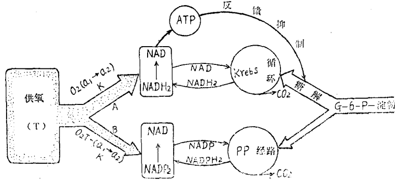
图4 野燕麦依靠EMP经路与PP经路平衡的发芽模式图 a 1 : 最大的氧消耗 a 2 : 有限的氧消耗 k: 氧气供应能力 T: 氧气供应量
