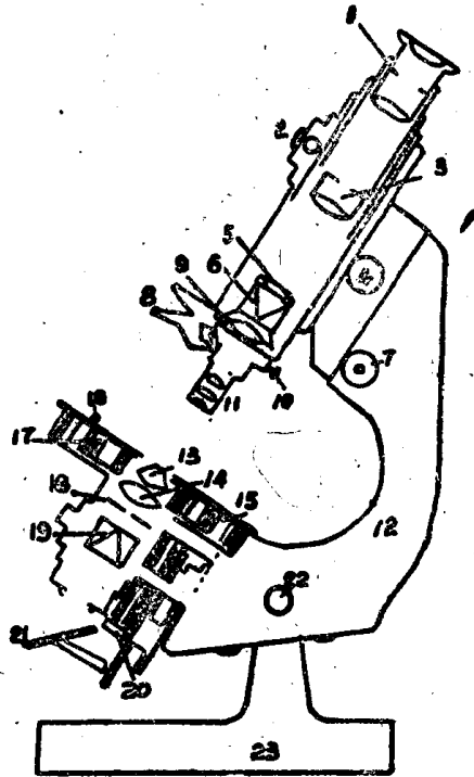
圖 1—1 偏光顯微鏡的構 造略圖
