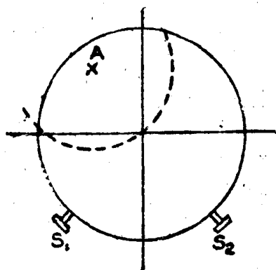
图 1—6 物镜的中心校正 S_1, S_2 是校正螺旋
