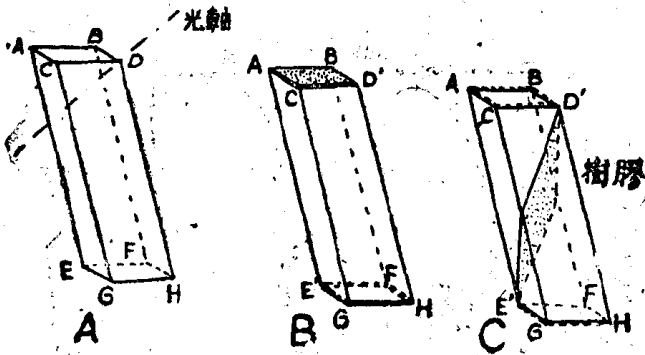
图 1—4 制造简单聶氏偏光鏡的步骤
