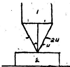
图 1-3 物镜对观察物体所形成的孔径角 1—物镜；2—光片
