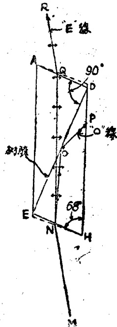
图 1-5 光通过哥氏偏光镜截面的途径
