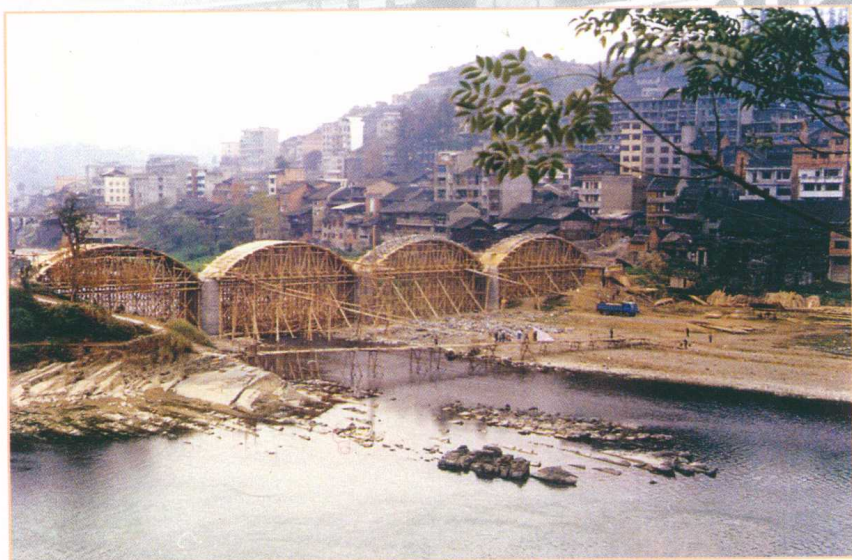
2001年12月6日，风雨桥四拱合拢(之一)
