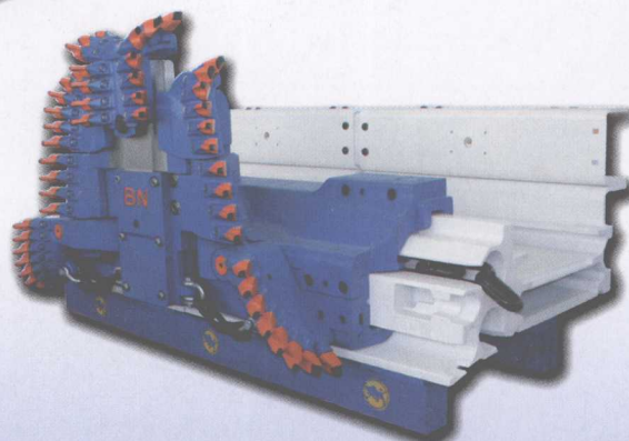
BH38/2×400 (315) 型刨煤机
