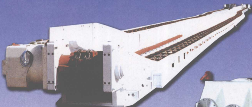
SGZ1000系列刮板输送机
