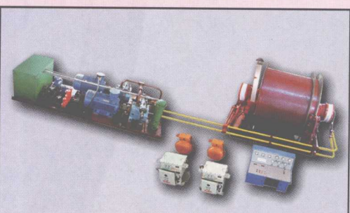
■ JKYB—2.0型液压防爆提升机
