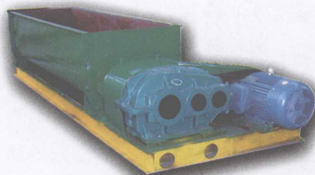
DJ370型单轴搅拌机
