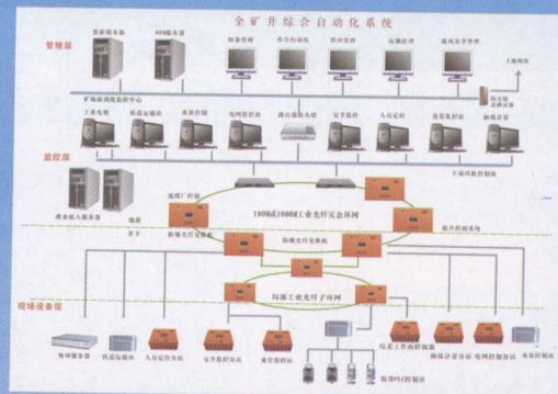
KJ90全矿井综合自动化监控系统
