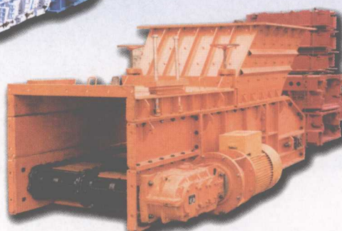
GLS750—1400系列链式给料机
