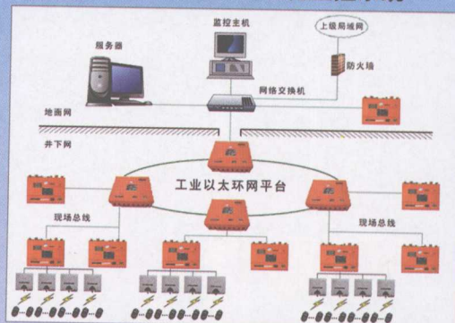
KJ251型煤矿人员管理系统
