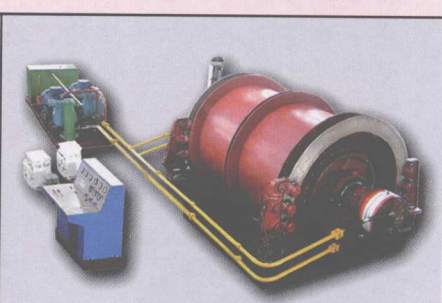
■ 2JKYB—3.5型液压防爆提升机
