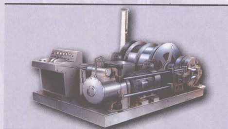
■ 2JTYB—1.2型液压防爆绞车
