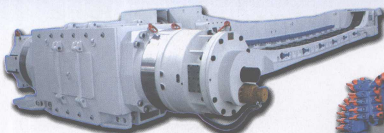
SGZ1000/3×855型刮板输送机
