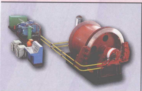
■ JKYB—3.0型液压防爆提升机
