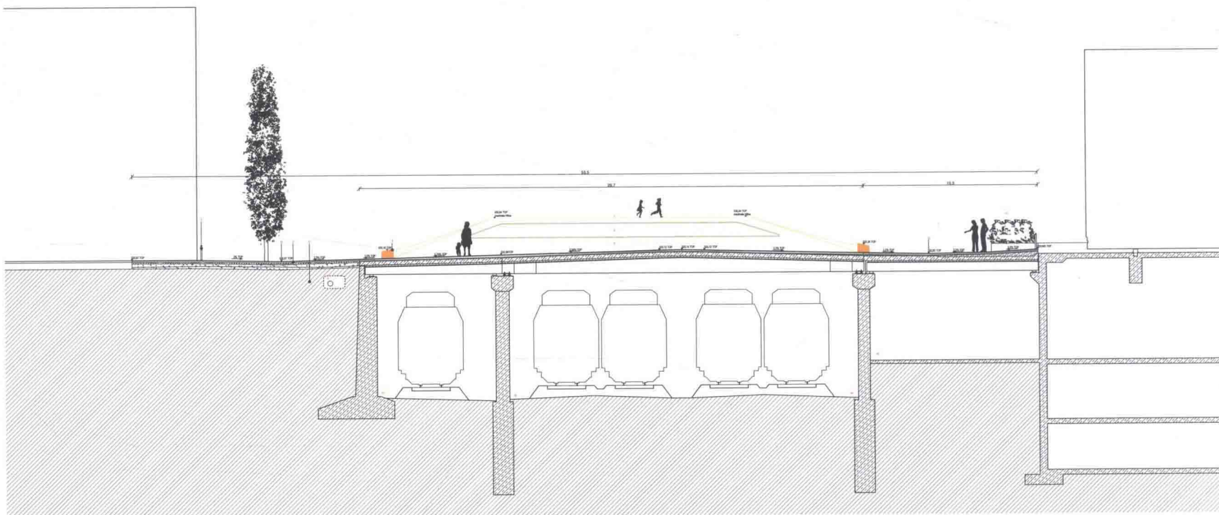
B02.5 Schemaquerschnitt Rasenhügel und Mauerband auf Brückenbauwerk
