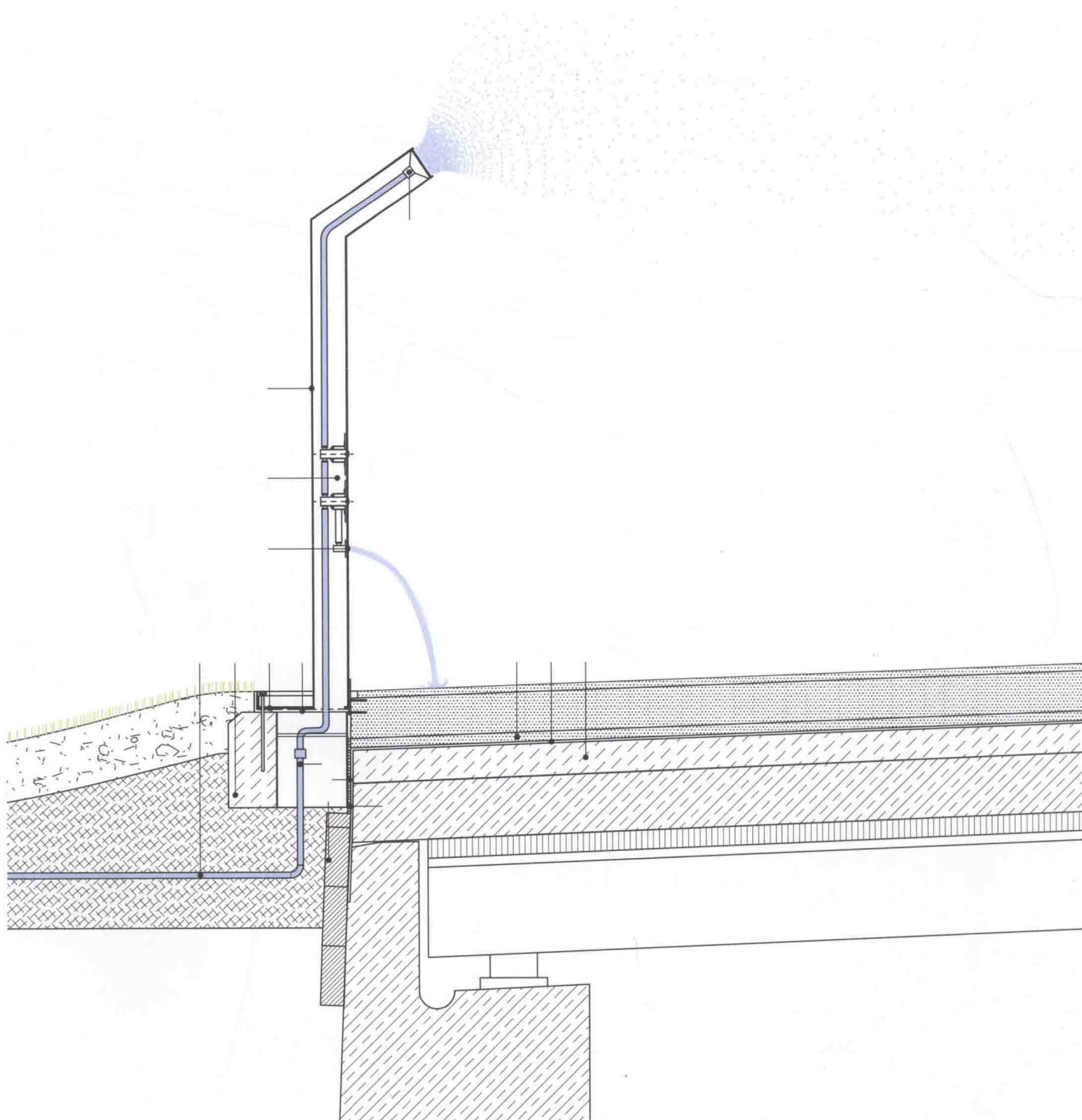
B11.4 - Schnitt Nebel- und Fußdusche
