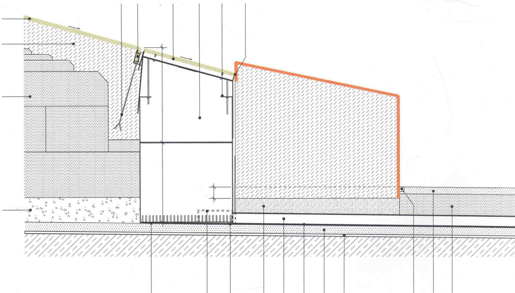
B05.5 - Regeldetail revisionskasten rasenhügel typ 1
